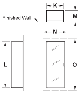
TRIMLESS
