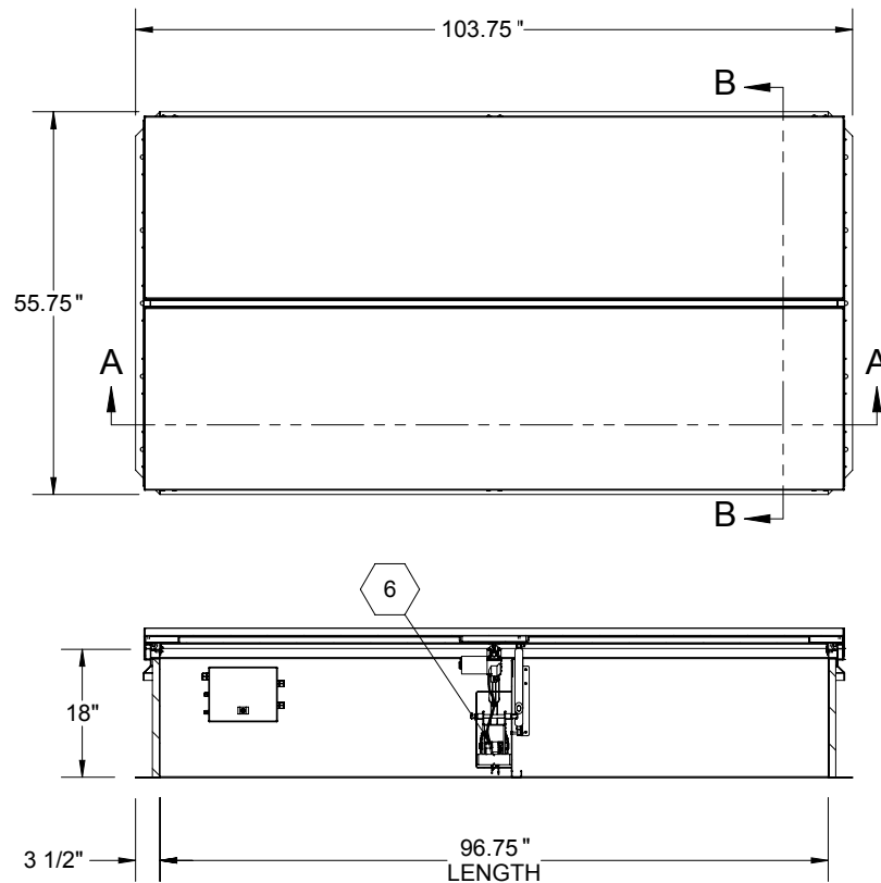
SECTION A-A
